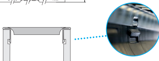
Fix-systeem
